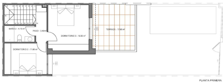
PLANTA PRIMERA
