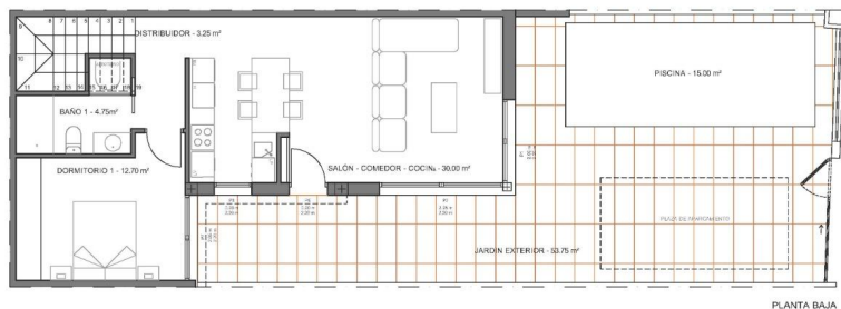
PLANTA BAJA
