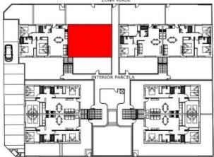
ESQUEMA PLANTA BAJA
