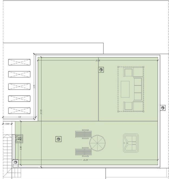
PLANTA CUBIERTA-SOLARIUM
