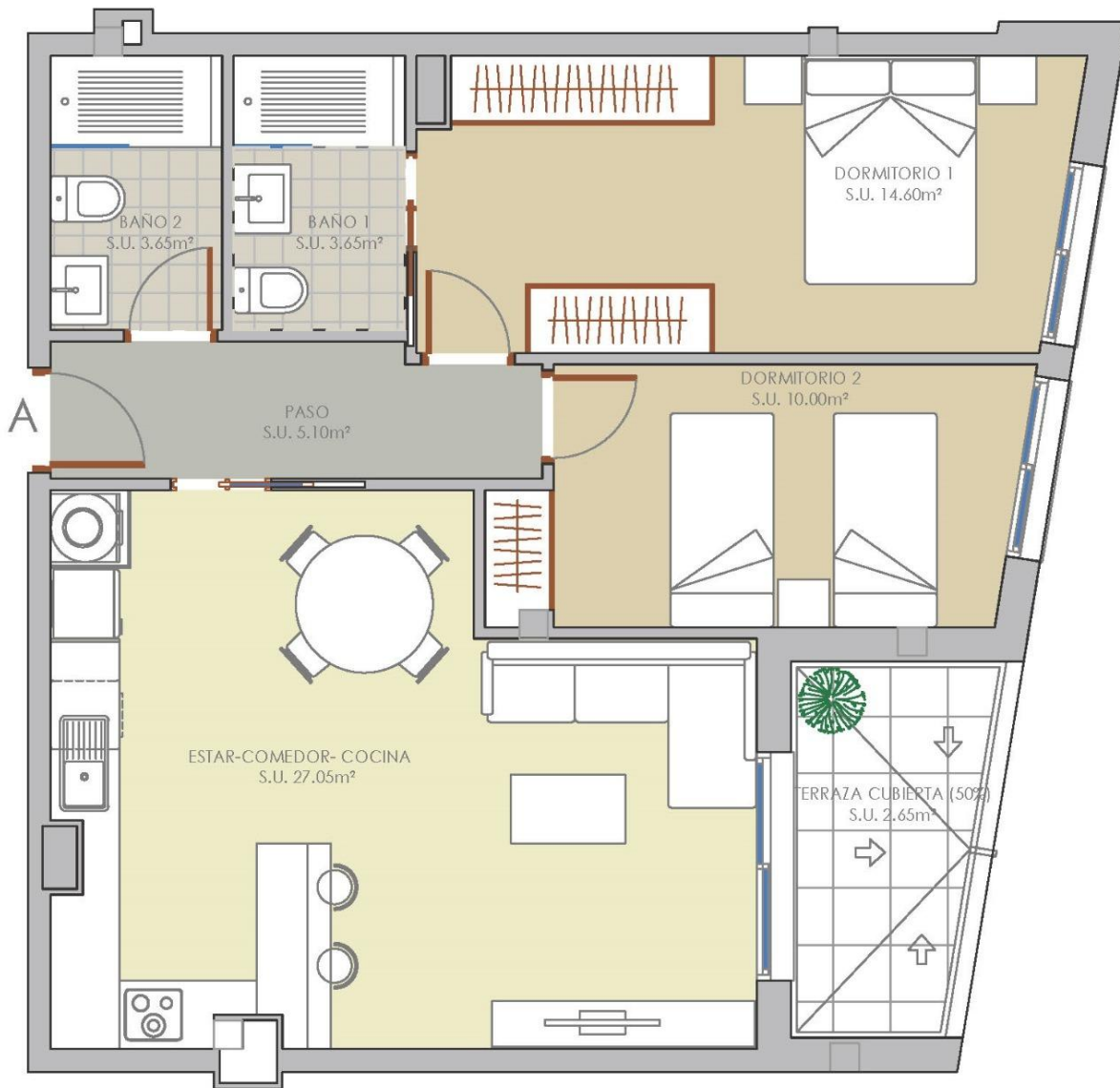
PLANTA 1º-2º-3º - A
