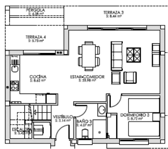
PLANTA BAJA
