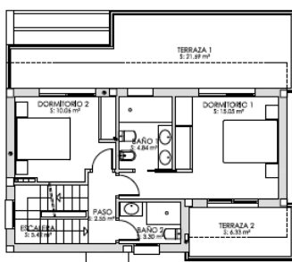
PLANTA ALTA
