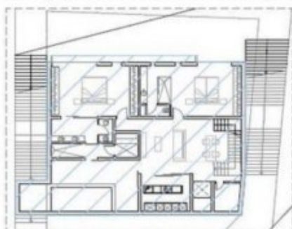
PLANTA SÓTANO
