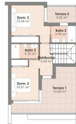
Planta Primera
