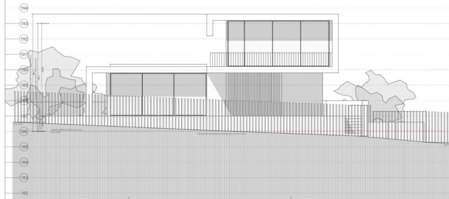
A.3.4 ALZADO Y SECCIONES A.3.4 SECCION D-D'
