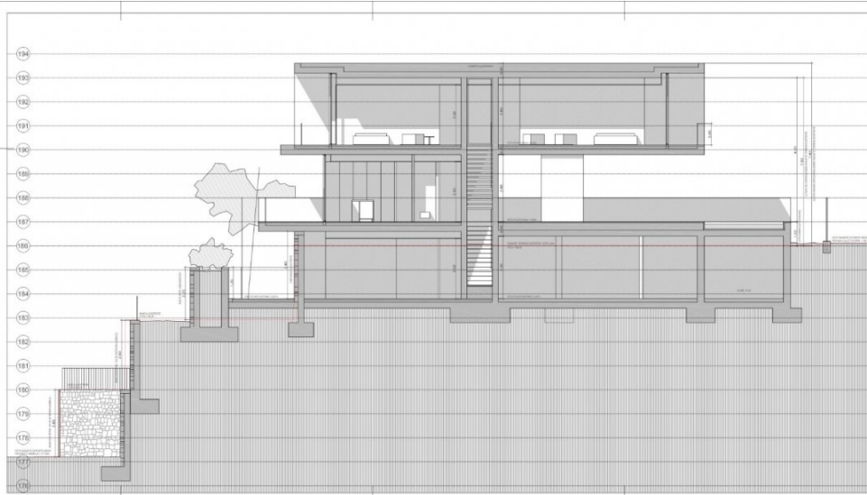
A.3.3 ALZADO Y SECCIONES A.3.3 SECCION C-C'
